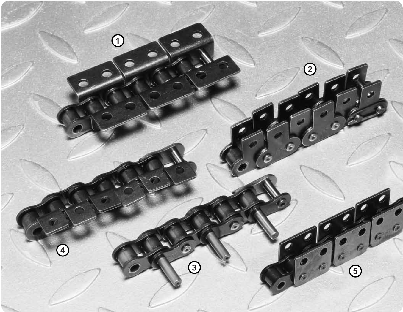
▲ 1 en 4 bevestigingslippen haaks 2 en 5 bevestigingslippen recht 3 verlengde pen
